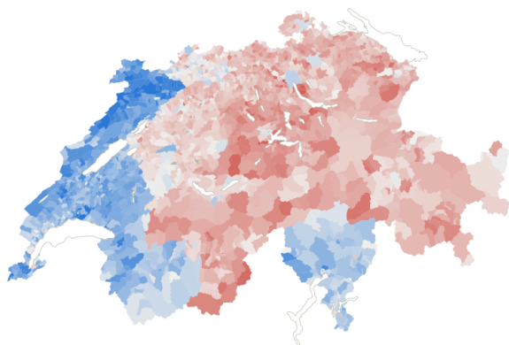
En rouge : droite
