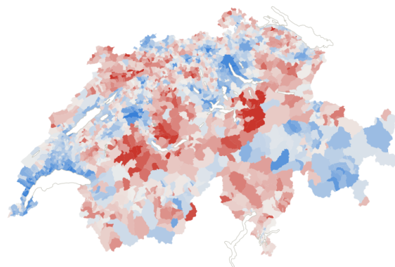
En rouge : souverainisme
