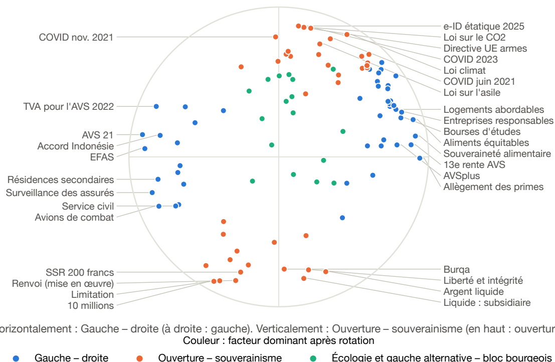
Fig. 10. – Les objets dans le plan tourné (corrélation de chaque objet avec F1 et F2). Couleur : le facteur auquel l'objet se rattache le plus, sur trois facteurs.
